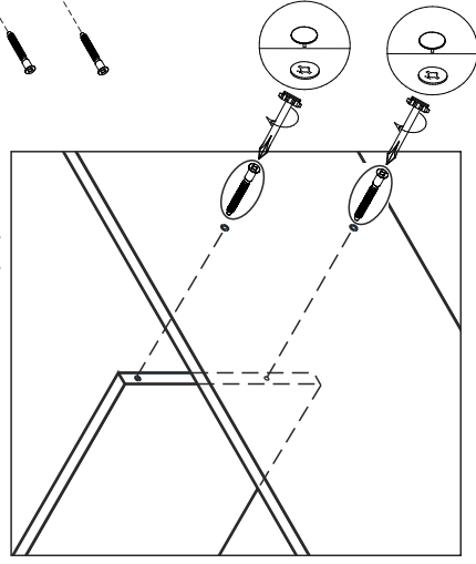
Крепление вязки к боковинам еврошурупами
